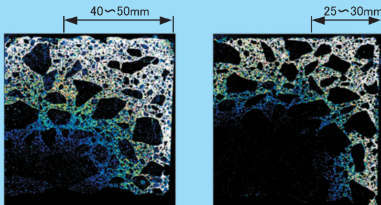
写真の見方 電子線マイクロアナライザーによる写真です。白っぽくなっている部分が塩素イオンの浸透を表します。
